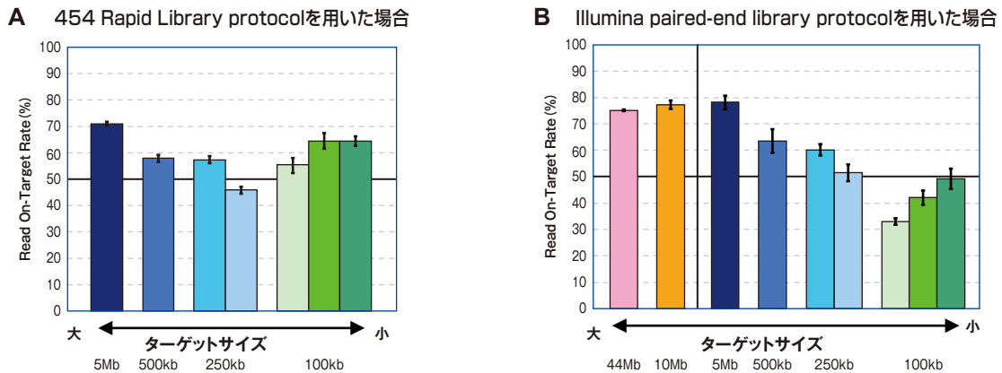
図2 SeqCap EZ Choiceを用いた場合のターゲットサイズとOn-Targetリードの割合 ターゲットサイズ、ターゲット領域の異なるデザインでSeqCap EZ Choiceを用いて、HapMapサンプルを(A)454 ゲノムシーケンサー、(B)Illumina GAllxでそれぞれシーケンスしました。キャプチャー&シーケンシング実験は独立して3回実施し、それぞれのデザインでのOn-Targetリード(%)の平均値(エラーバーは±1 SD)を表示しています。
