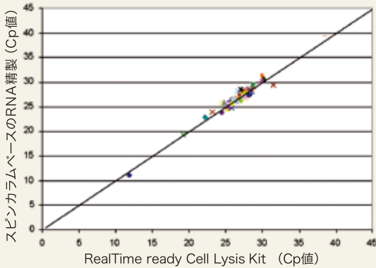
図2: スピンカラム法による定量PCRの結果との高い相関 19種類のリファレンス遺伝子について2種類のワークフローでのリアルタイムPCRの結果(Cp値)を比較。 (サンプル:30,000個のHela細胞)
