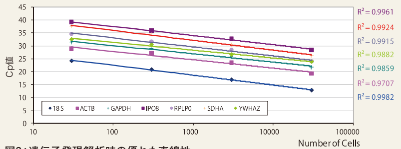
図3: 遺伝子発現解析時の優れた直線性 7種類のターゲット遺伝子の、4桁の細胞使用量における直線性。 (サンプル:30~30,000個のMCF-7細胞)
